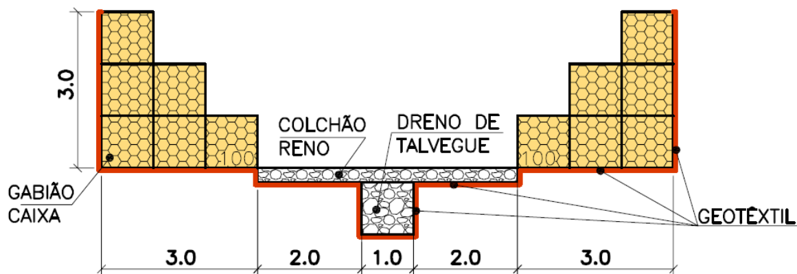
Figura 5. Seção transversal do canal.
