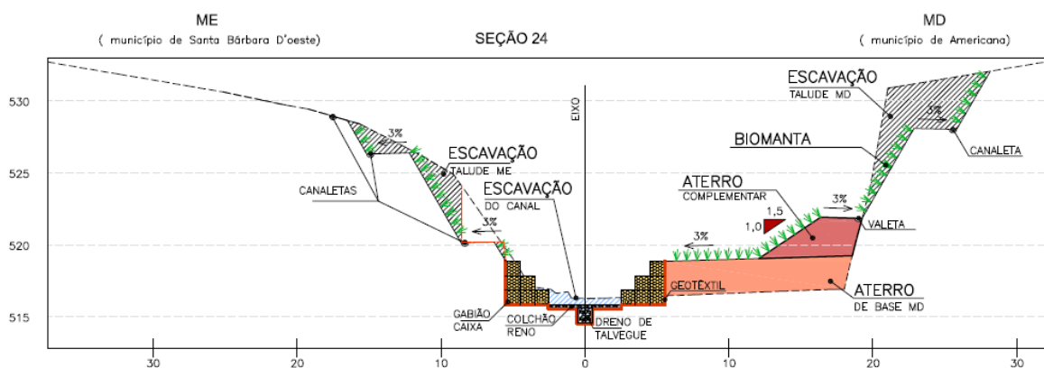
Figura 8. Seção 24 – Canal, cortes e aterros de base.
