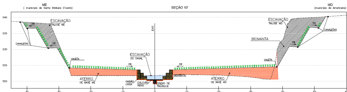
Figura 7. Seção 17 – Canal, cortes e aterros de base.
