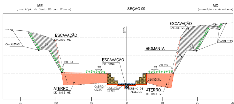
Figura 6. Seção 9 – Canal, cortes e aterros de base.
